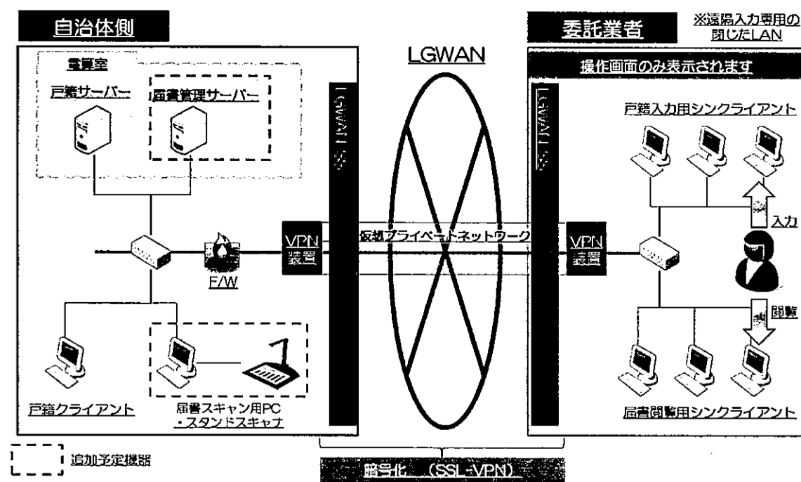
ネットワーク概要図
