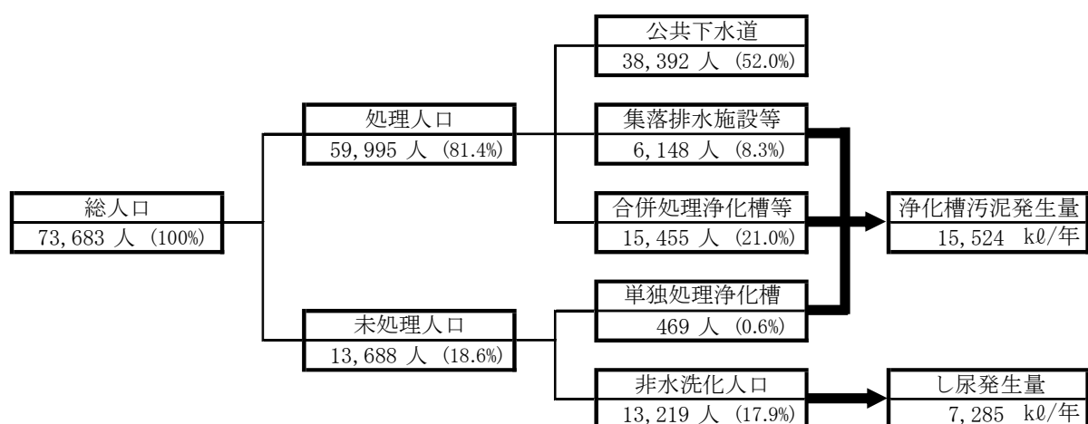
図 7-1-4 計画区域の生活排水処理状況（令和 6 年度 第 1 中間目標）
