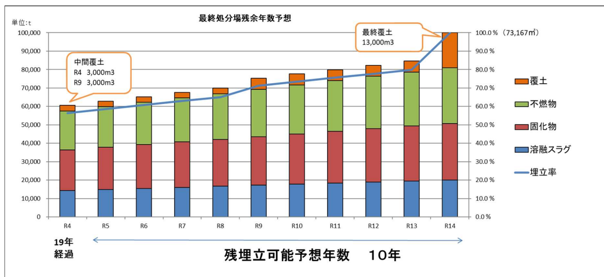
図 4-2-1 最終処分場埋立計画
