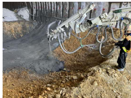
写真 トンネル吹付状況
