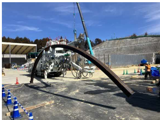
写真 トンネル使用機械
