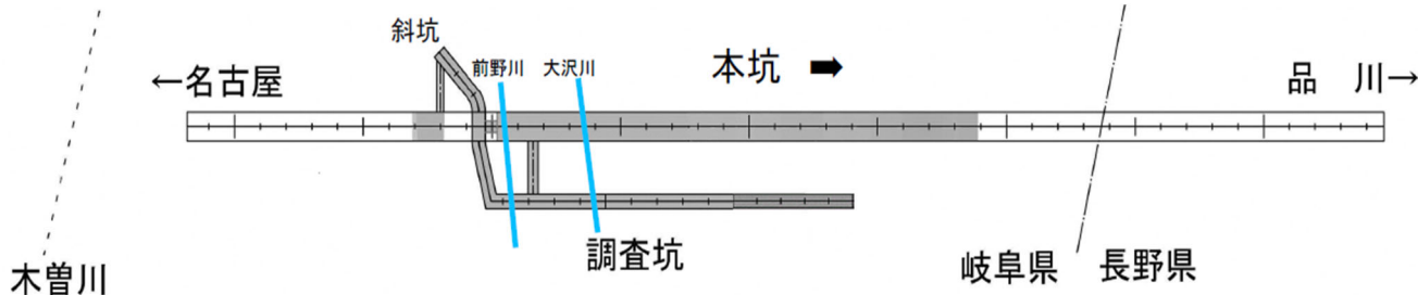
路盤・覆工状況
