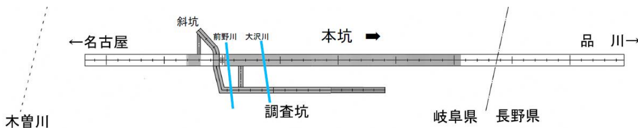
覆工コンクリート工事
