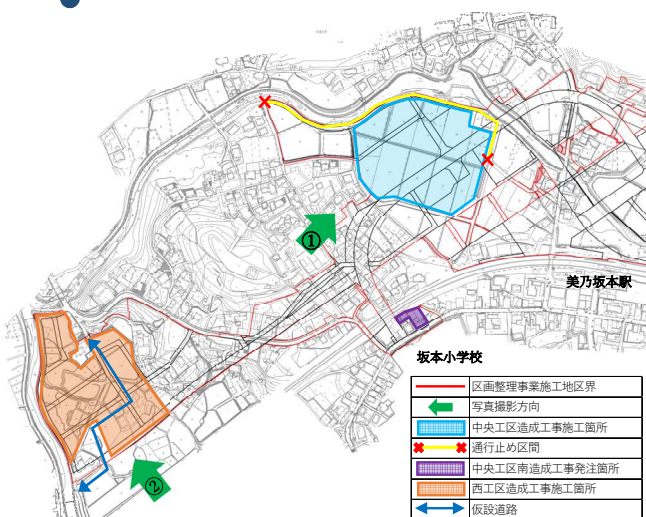
【工事状況概要図】
