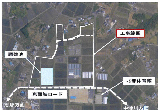
本工事の工事範囲
