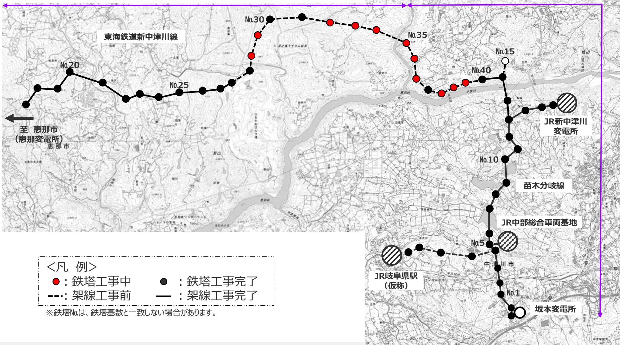
リニア関連送電線新設工事（3工区）
