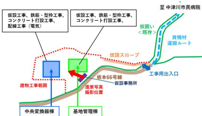
建物工事範囲 概要図
