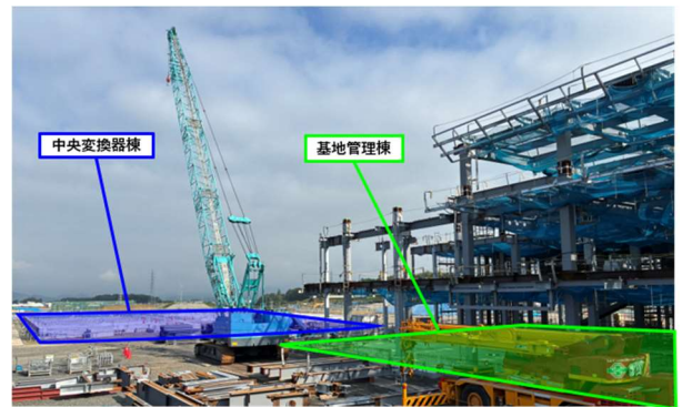
建物工事範囲 遠景写真 （撮影位置は左図をご参照ください）
