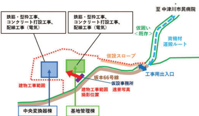
建物工事範囲 概要図
