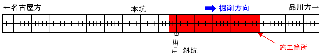
図-1 トンネル掘削進捗平面図（模式図）
