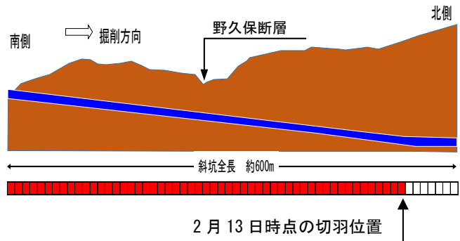
図-1 トンネル掘削進捗縦断面図
