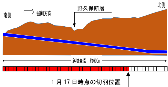
図-1 トンネル掘削進捗縦断図
