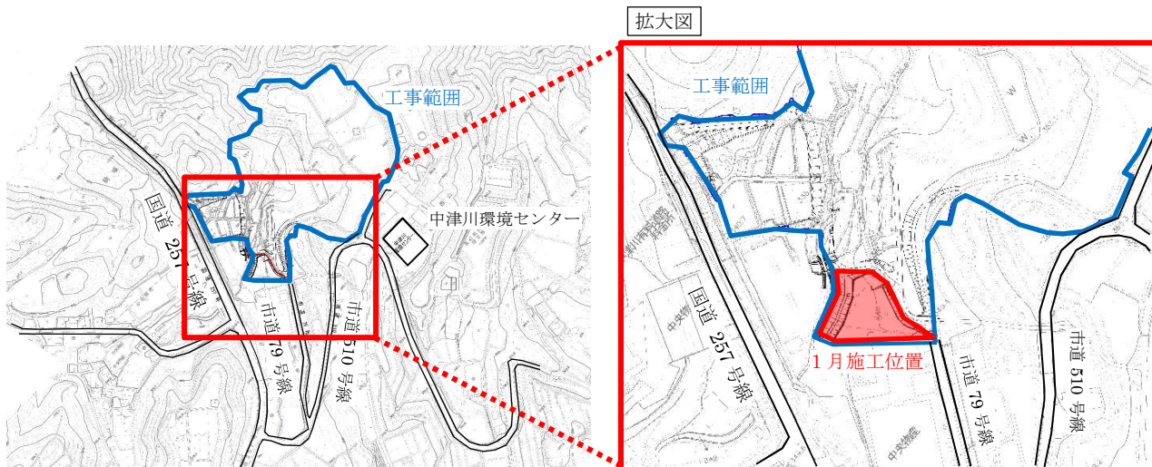
図1 工事範囲図
