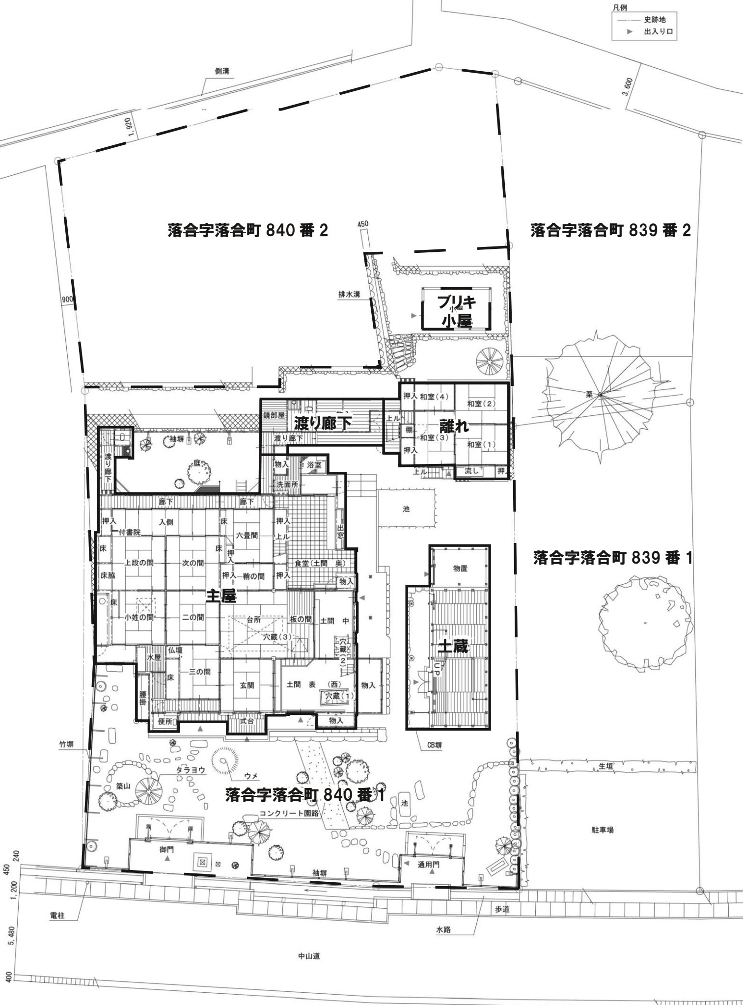
図 3 全体配置図
