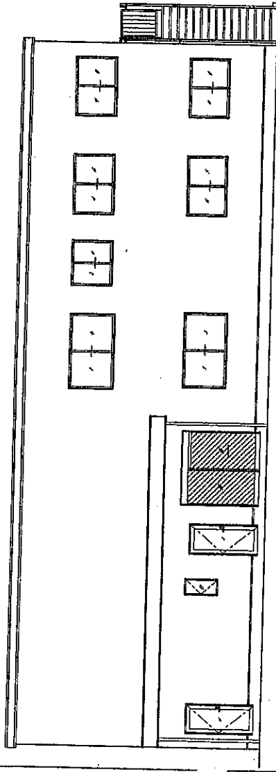
【 西側立面図 S=1/100 】
