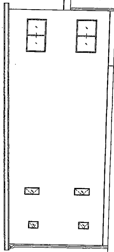
【 北側立面図 S=1/100 】
