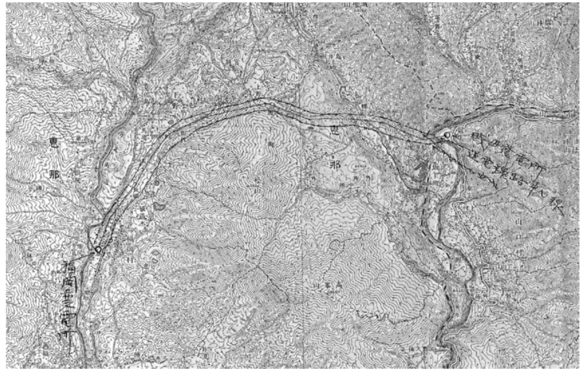
← 賤母発電所から福岡駅までの送電線路図(市史編集室)
