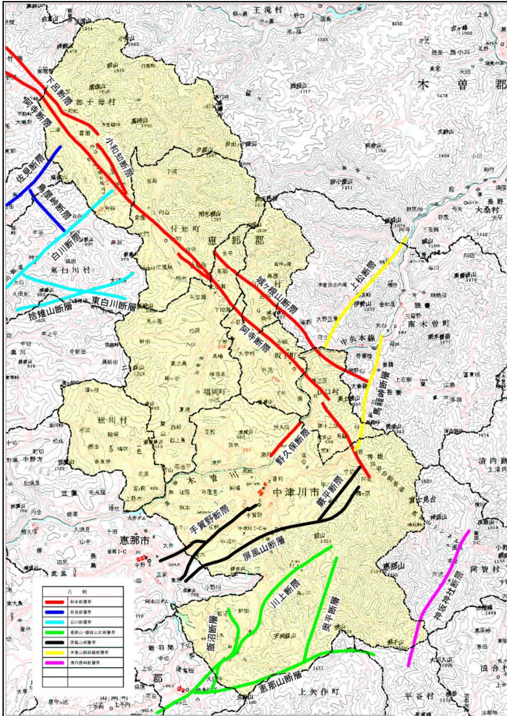
〔中津川市周辺の活断層〕
